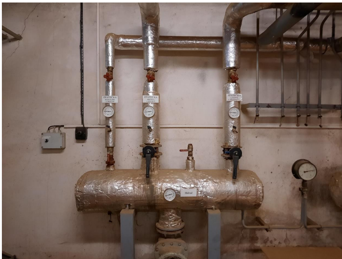
Foto č. 3 – sběrač před předávací stanicí
