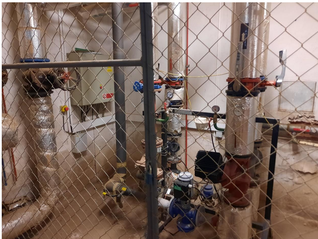
Foto č. 2 – rozdělovač před předávací stanicí
