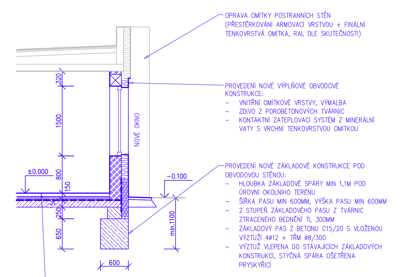
Řez A-A
