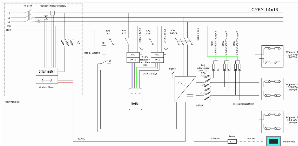
Obr. 34: Blokové schéma FVe. [zdroj: PD – FVe]
