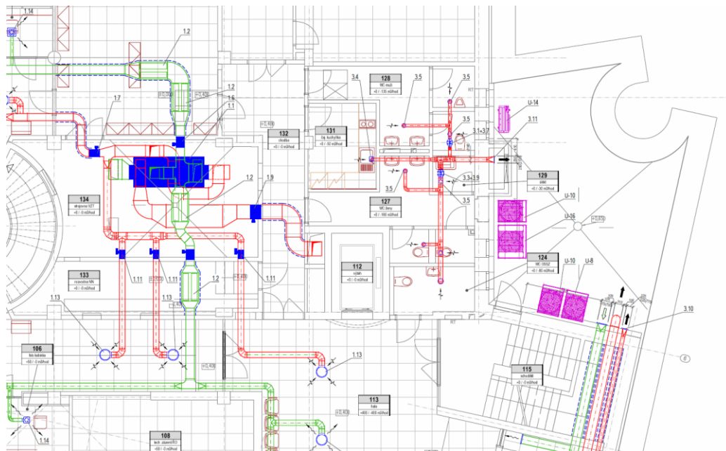
Obr. 31: Půdorys střechy 1.NP – vzduchotechnika a chlazení. [zdroj: PD – VZT+CH]
